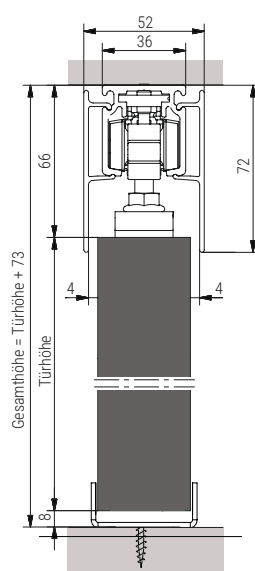
FLOW Deckenmontage
