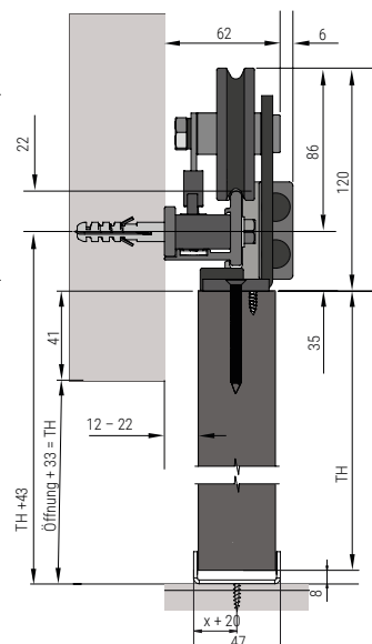
SHIFT Wandmontage
